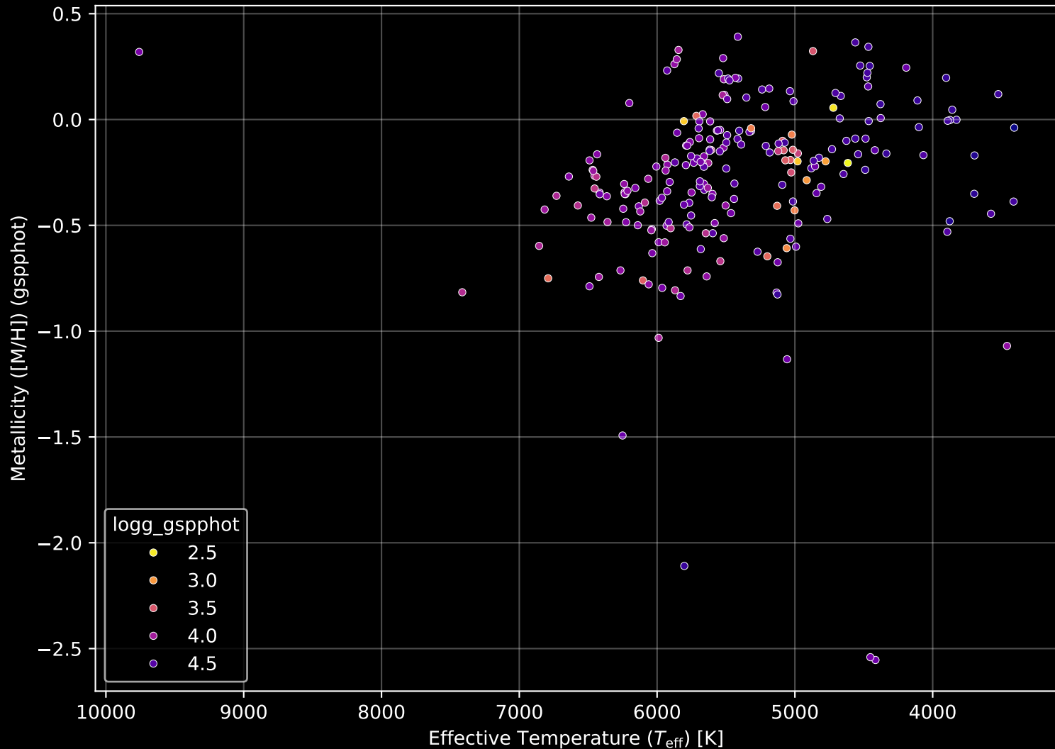
APOGEE DR17 Field: [180-60] Stellar Population Parameters (n= 228)
